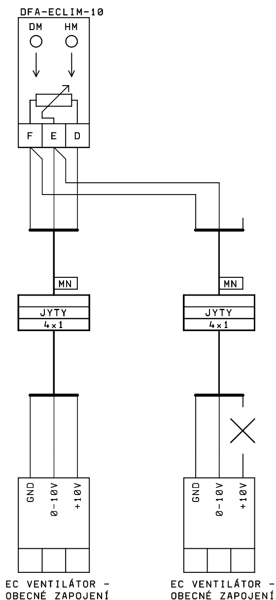
DVA EC MOTORY REGULOVANÉ VE STEJNÉM ROZSAHU NAPĚTÍ
