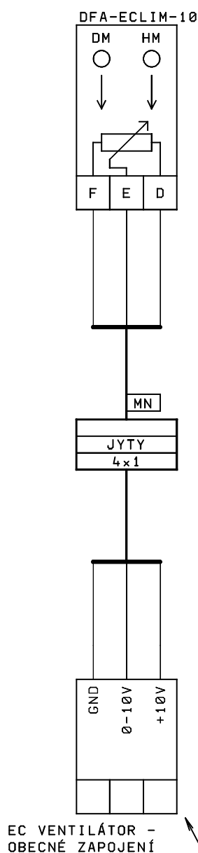
JEDEN EC MOTOR
